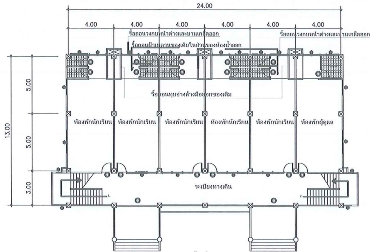
แปลนพื้นชั้นล่าง (เดิม)
