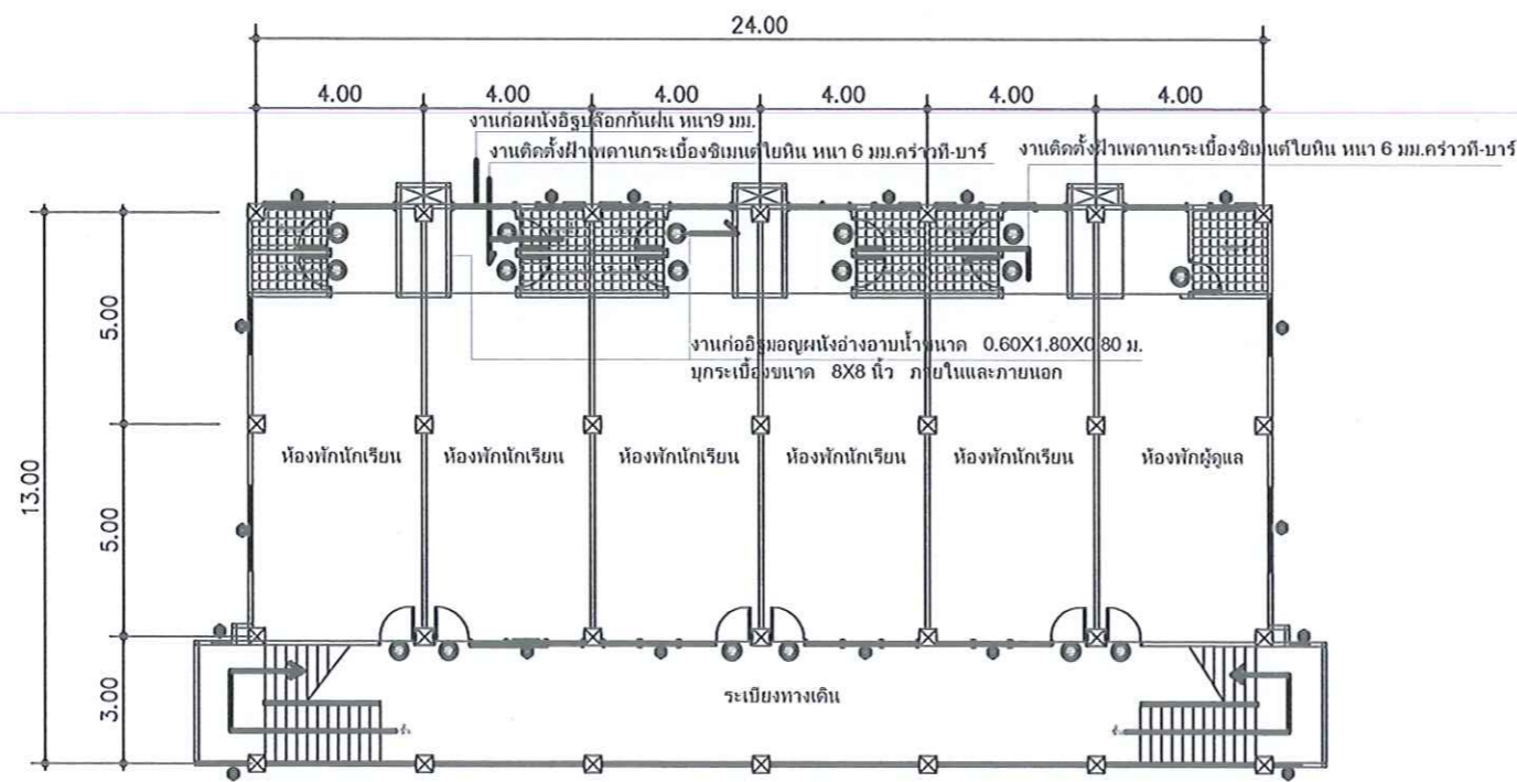
แปลนพื้นที่ชั้น 2,3,4 (เดิม)
