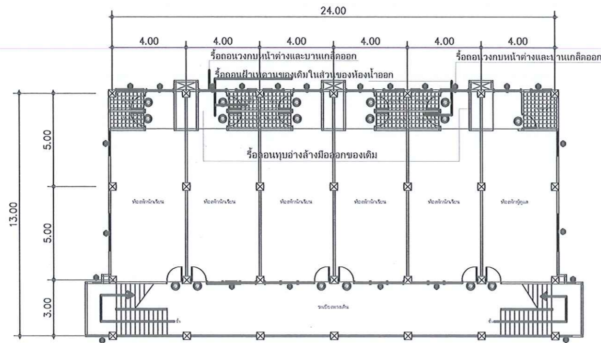
แปลนพื้นชั้น 2,3,4 (เดิม)
