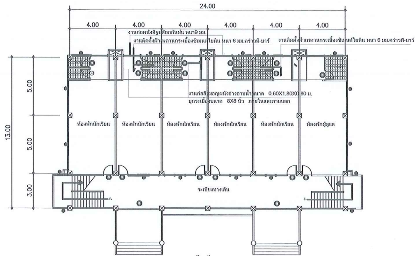
แปลนพื้นที่ชั้นล่าง (เดิม)
